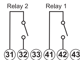
Abb. 27 Relaisausgang
