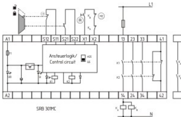
Schaltungsbeispiel
